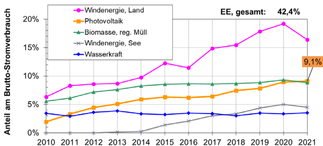
Abbildung 3: Entwicklung des Anteils Erneuerbarer Energien am Bruttostromverbrauch in Deutschland, Daten aus [BMWi1], [BDEW3]
