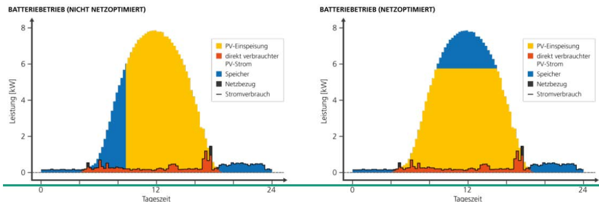
Abbildung 57: Gegenüberstellung der konventionellen und der netzdienlichen Betriebsführung [ISE7]
