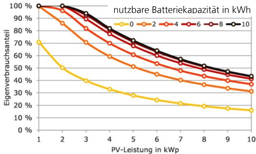
Abbildung 56: Eigenverbrauchsanteil in Abhängigkeit von Batteriekapazität und Leistung des Solargenerators für einen Einfamilienhaushalt mit einem Jahresstromverbrauch von 4.700 kWh. [Quasch]
