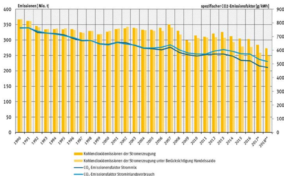
Abbildung 41: Spezifische und absolute CO 2 -Emissionen der Stromerzeugung in Deutschland [UBA6]
