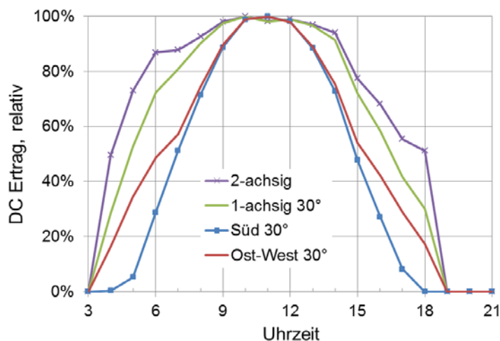
Abbildung 52: Stromertragsprofile von PV-Anlagen in verschiedenen Montagevarianten, berechnet mit der Software PVsol für einen überwiegend klaren Julitag am Standort Freiburg
