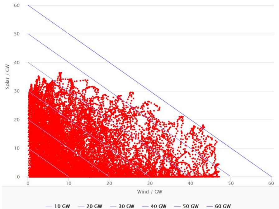
Abbildung 25: Mittlere Leistung für die Einspeisung von Sonnen- und Windstrom im Jahr 2021, 15-Minuten-Werte [ISE4]
