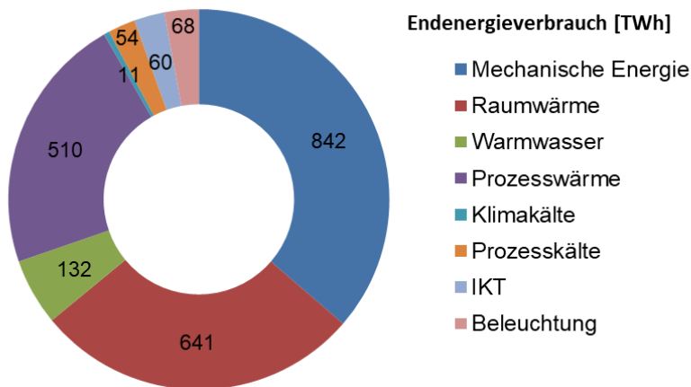
Abbildung 47: Struktur des Endenergieverbrauchs nach Anwendungsbereichen für Deutschland im Jahr 2020, Zahlen aus [BMWi1]
