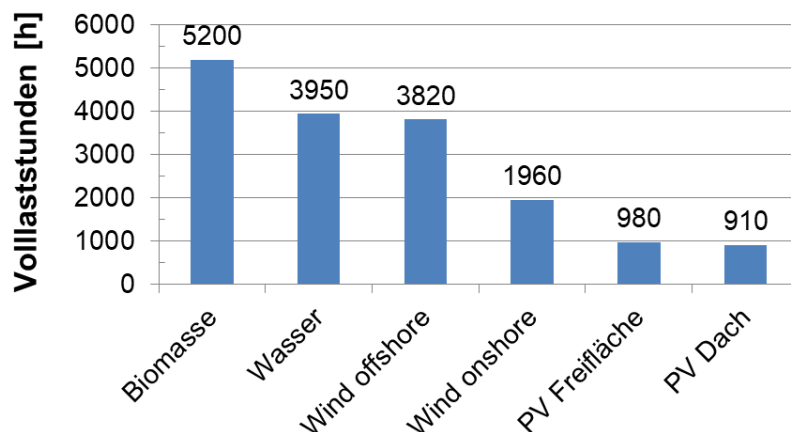
Abbildung 35: Prognostizierte Vollbenutzungsstunden für Stromerzeugung aus EE, Daten aus [ÜNB1]
