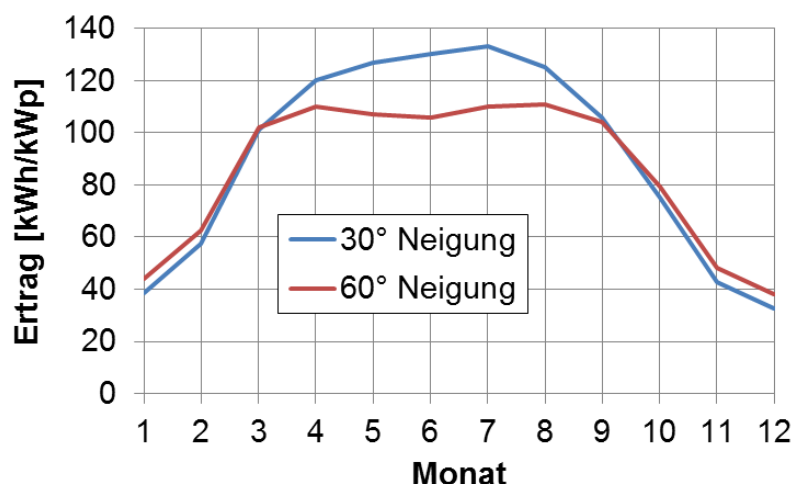
Abbildung 53: Rechenbeispiel für den spezifischen Monatsertrag einer PV-Anlage am Standort Freiburg für südorientierte Module mit 30° Neigung (max. Jahresertrag) und 60° Neigung
