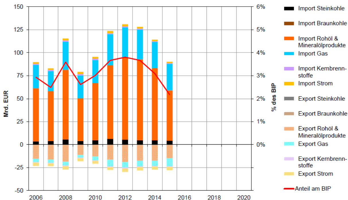
Abbildung 46: Entwicklung der Kosten für die Bereitstellung der Primärenergie in Deutschland [ÖKO3]
