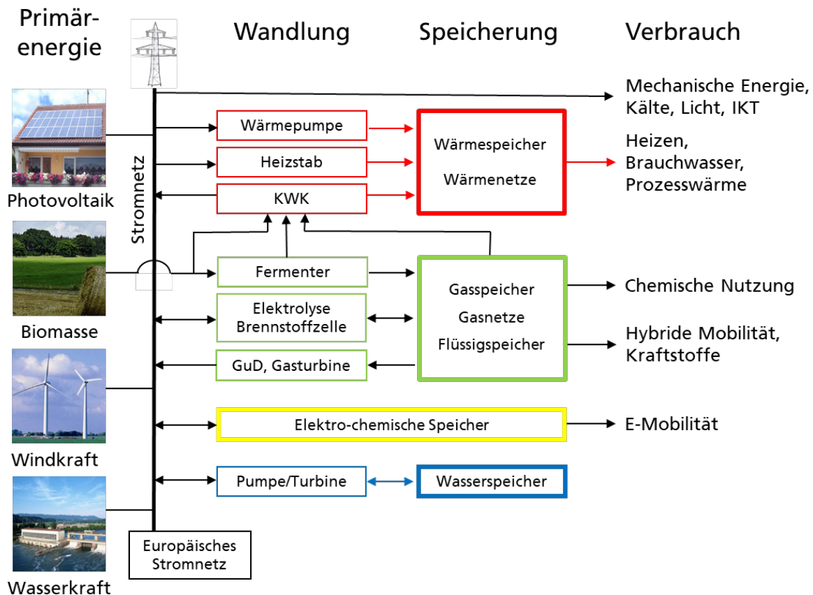
Abbildung 62: Vereinfachte schematische Darstellung eines Erneuerbaren Energiesystems mit den wichtigsten stromnetzgebundenen Bausteinen der Gewinnung, Wandlung, Speicherung und des Verbrauchs; IKT: Informations- und Kommunikationstechnik, KWK: Kraft-Wärme-Kopplung, GuD: Gas-und-Dampf-Kombikraftwerk
