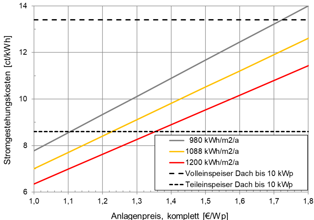
Abbildung 18: Abschätzung der Stromgestehungskosten für kleine PV-Anlagen unter verschiedenen Einstrahlungsbedingungen, dazu Vergütungen gemäß [EEG2023]
