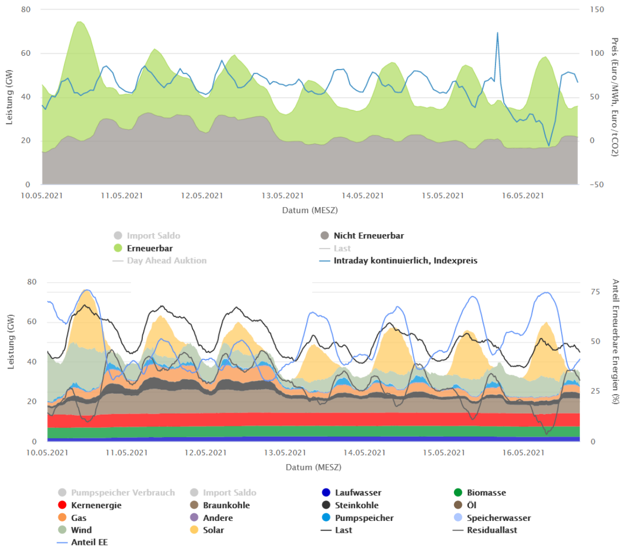
Abbildung 27: Beispiel für den Verlauf von Börsenstrompreisen, konventioneller und regenerativer Stromerzeugung der 19. Kalenderwoche im Mai 2021 [ISE4]
