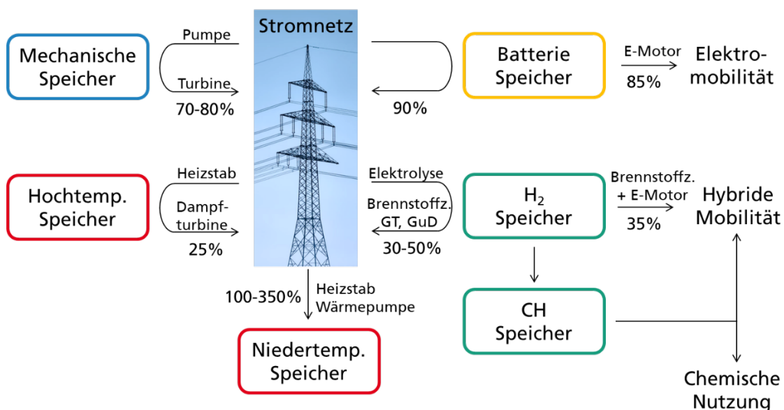
Abbildung 59: Technologien für Energiespeicher und -wandler mit heute erzielbaren Wirkungsgraden am Ende der Wandlerkette, ohne Kraft-Wärme-Kopplung (GT: Gasturbine, GuD: Gas- und Dampfturbine)
