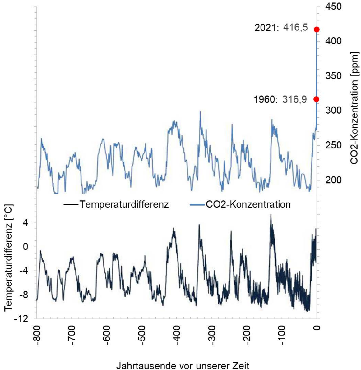
Abbildung 38: Schätzungen der atmosphärischen CO 2 -Konzentration und der Temperaturdifferenz in der Antarktis auf Basis von Eisbohrkernen [EPA]; Rot: zwei neuere CO 2 -Messwerte des Mauna Loa Observatory [ https://www.esrl.noaa.gov/gmd/ccgg/trends/data.html ]
