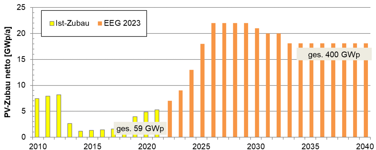
Abbildung 2: Netto-PV-Zubau: Ist-Werte bis 2021, möglicher Ausbaupfad zur Erreichung der gesetzlichen Ziele [EEG2023].
