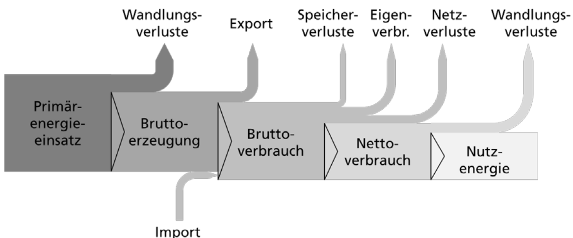
Abbildung 64: Begriffe der Stromerzeugung und des -verbrauchs
