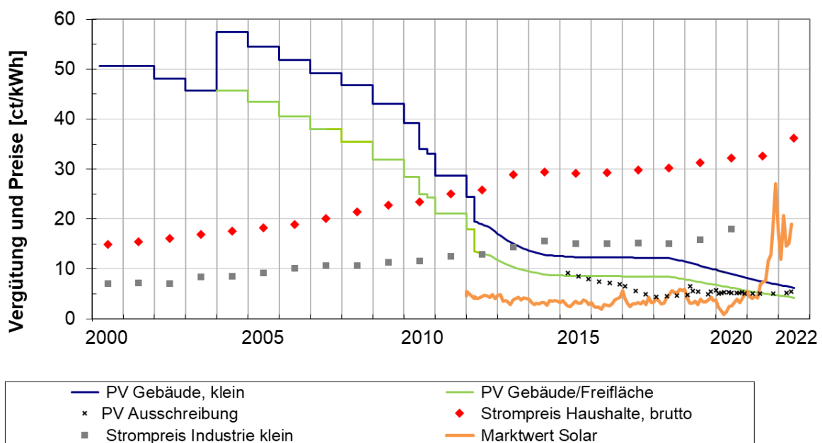
Abbildung 6: EEG-Vergütung für PV-Strom nach dem Datum der Inbetriebnahme des Kraftwerks, mittlere Vergütung in den Ausschreibungen der Bundesnetzagentur, Strompreise, Marktwert Solarstrom, Daten aus [BMW1], [BDEW1], [NETZ]
