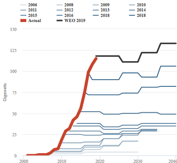
Abbildung 51: IEA-Prognosen seit 2006 und tatsächliche Entwicklung des globalen jährlichen PV-Zubaus [Carb]
