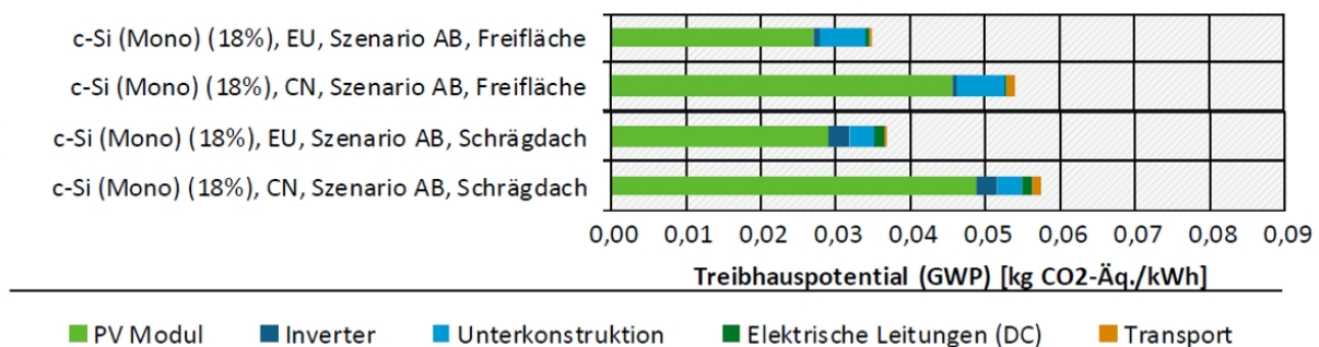
Abbildung 39: Treibhauspotenzial der Stromerzeugung mit mono c-Si PV für Dach- und Freiflächenanlagen [UBA7]
