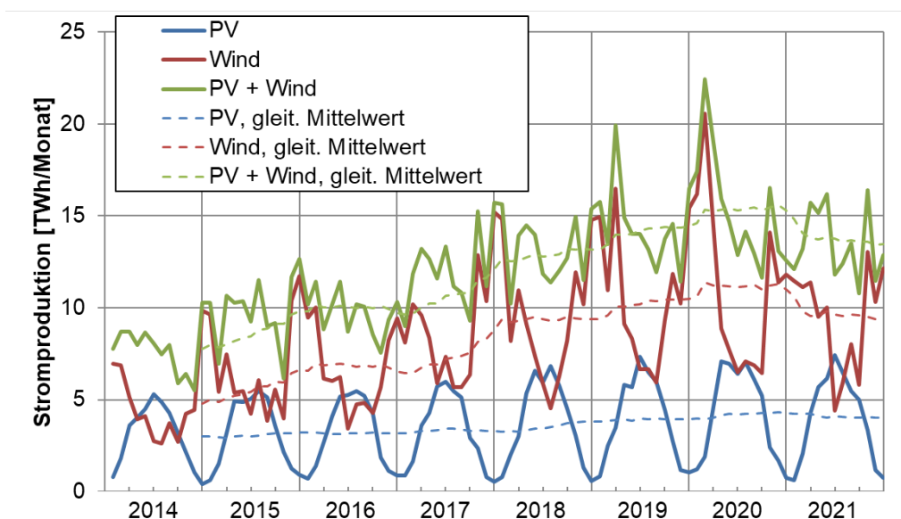
Abbildung 26: Monatssummen PV- und Windstromproduktion, Daten aus [ISE4]
