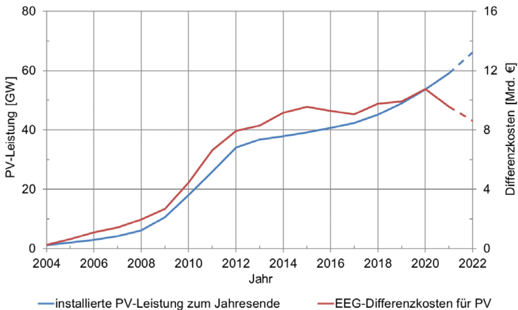
Abbildung 10: PV-Ausbau und Vergütungssumme, Daten aus [BMWi1], [BMWK3]
