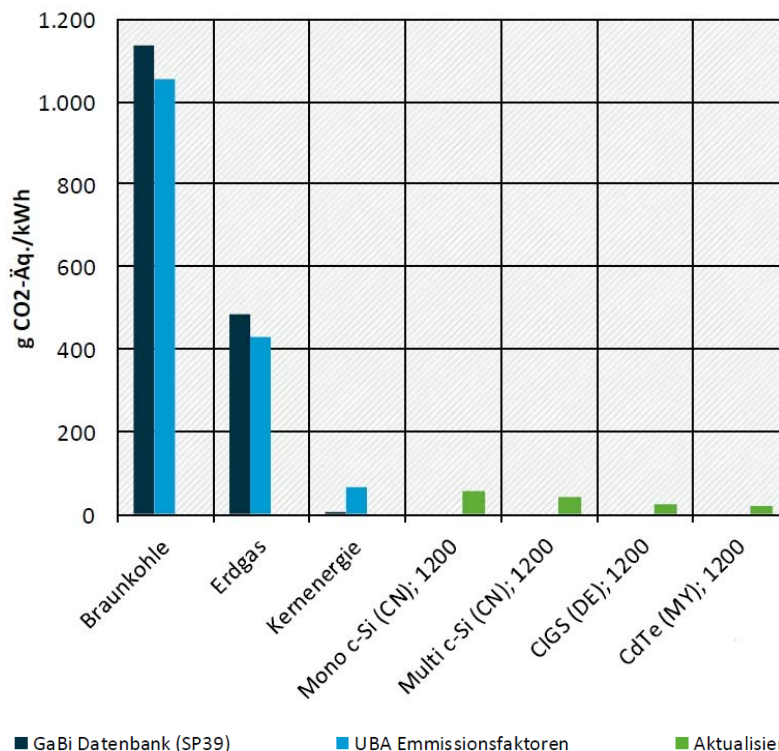
Abbildung 40: Treibhauspotenzial verschiedener Stromerzeugungstechnologien [UBA7]
