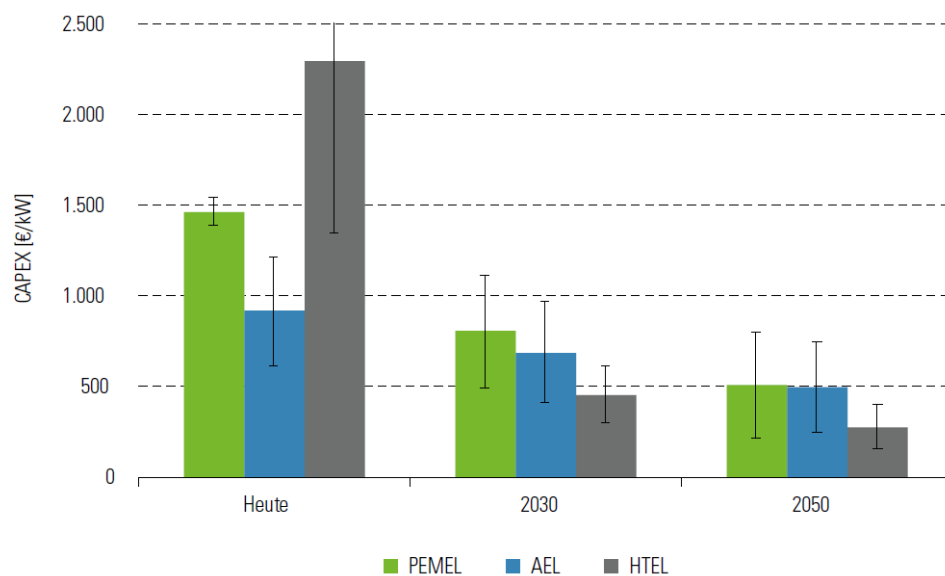
Abbildung 58: Spezifische Investitionskosten für verschiedene Elektrolyseurtechnologien (PEMEL: Membranelektrolyse, AEL: Alkalische Elektrolyse, HTEL: Hochtemperatur-Elektrolyse, [NOW])
