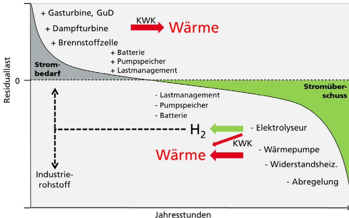
Abbildung 49: Schematische Darstellung einer Residuallastkurve für Deutschland bei Stromversorgung mit 100 % EE, mit Erzeugern (+) und Lasten (-)
