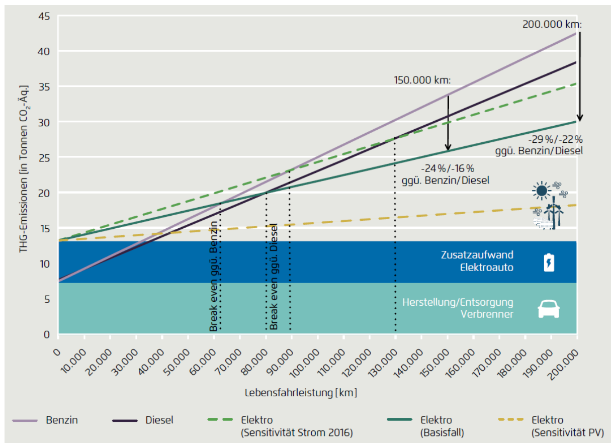
Abbildung 55: Treibhausgasemissionen von heutigen Fahrzeugen der Kompaktklasse in Abhängigkeit von der Fahrleistung [AGORA1]
