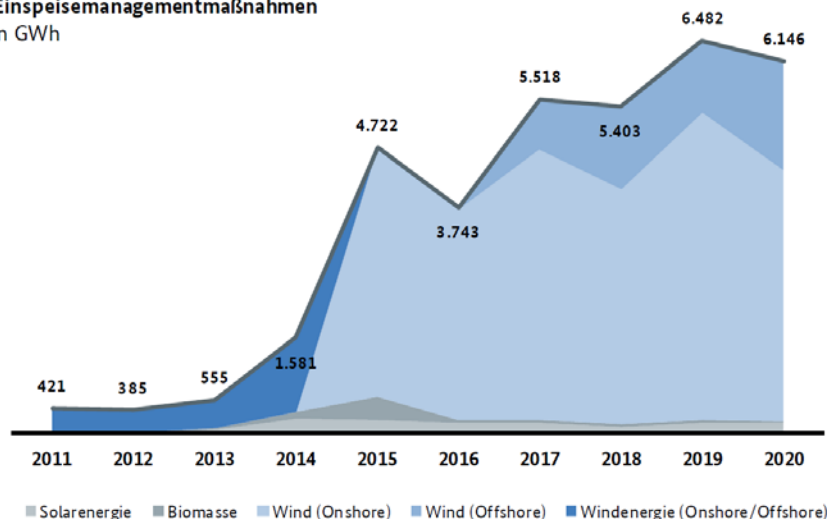
Abbildung 23: Abgeregelte elektrische Energie [BNA2]
