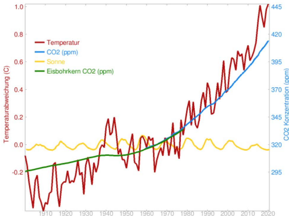
Abbildung 37: Entwicklung der atmosphärischen CO 2 -Konzentration, der mittleren globalen Temperaturveränderung und der Sonnenaktivität ( http://herdsoft.com/climate/widget/ ).
